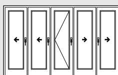
Схема 532 4 складывающиеся сдвижные створки 1 поворотная створка
