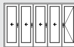
Схема 541 [1] 4 складывающиеся сдвижные створки 1 поворотная створка
