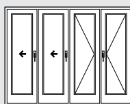
Схема 431 [1] 2 складывающиеся сдвижные створки 1 ступельная поворотная створка, 1 поворотная створка
