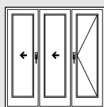
Схема 321 [1] 2 складывающиеся сдвижные створки 1 поворотная створка
